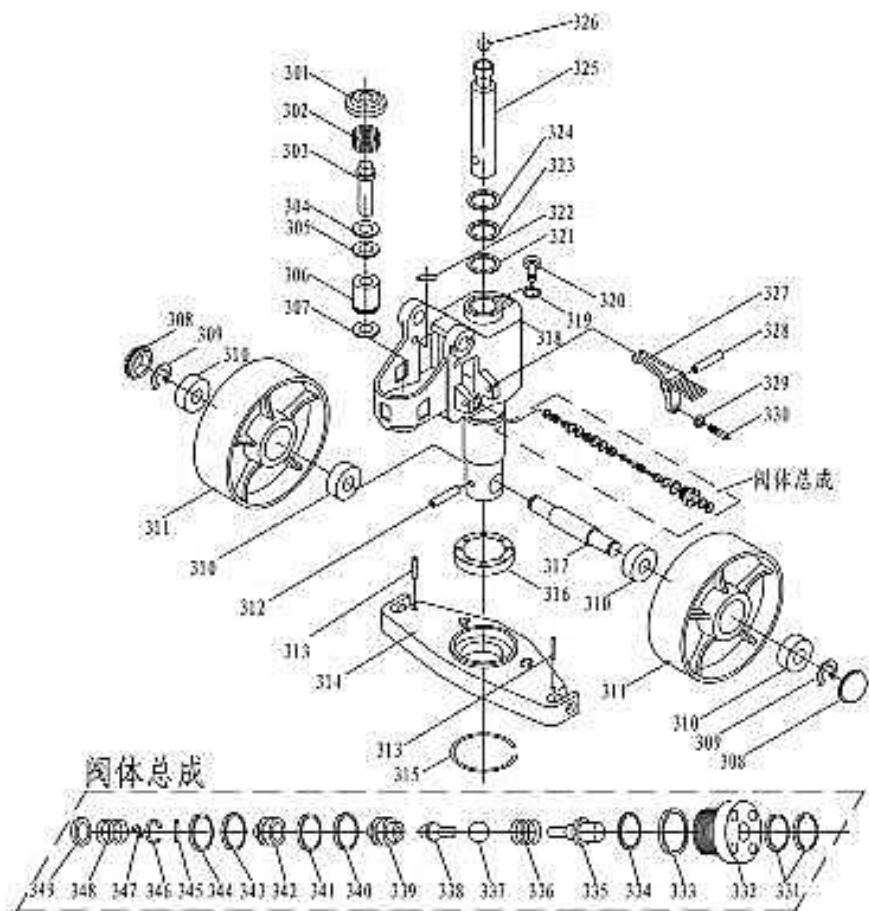
Рисунок 7. Взрыв-схема гидроузла тележки АС.
